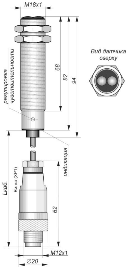
Габаритный чертеж
