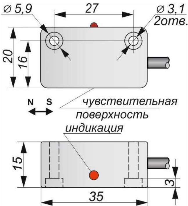
Габаритный чертеж
