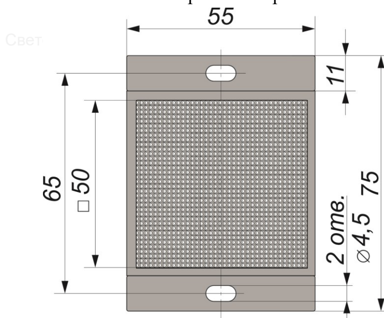
Габаритный чертеж
