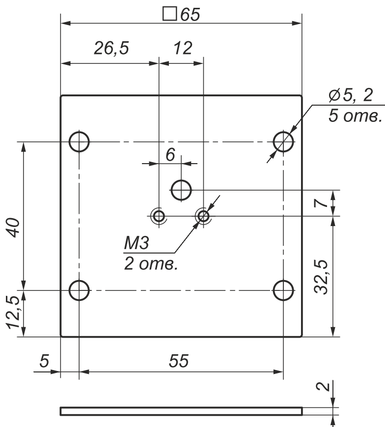
Габаритный чертеж
