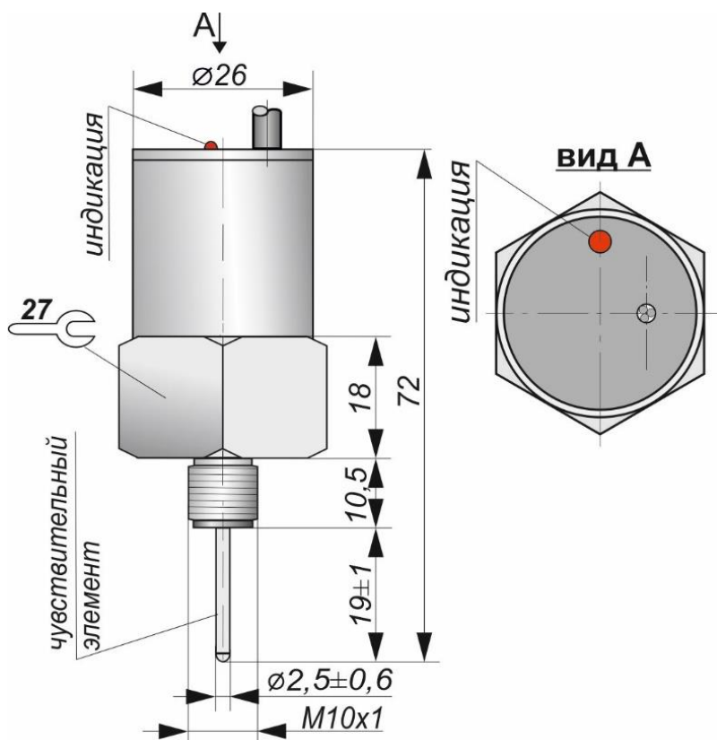
Габаритный чертеж
