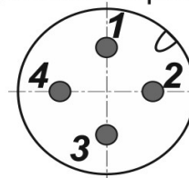
Цоколевка разъема
