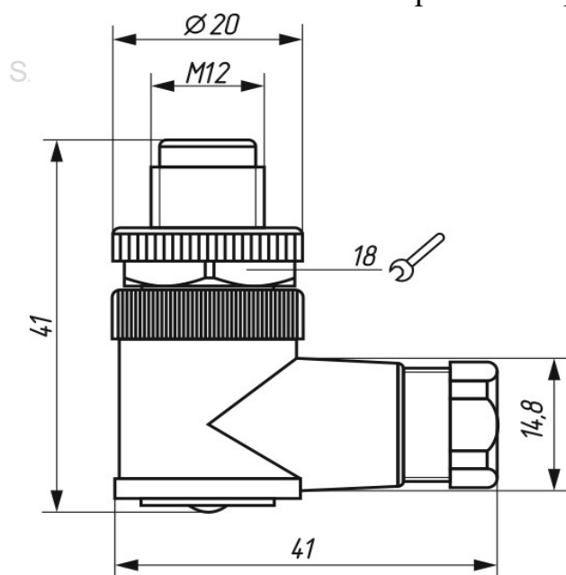
Габаритный чертеж
