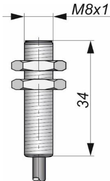
Габаритный чертеж
