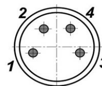
Цоколевка разъема
