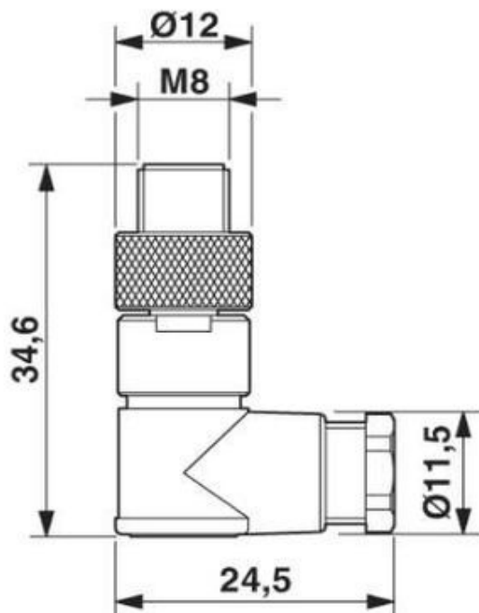
Габаритный чертеж
