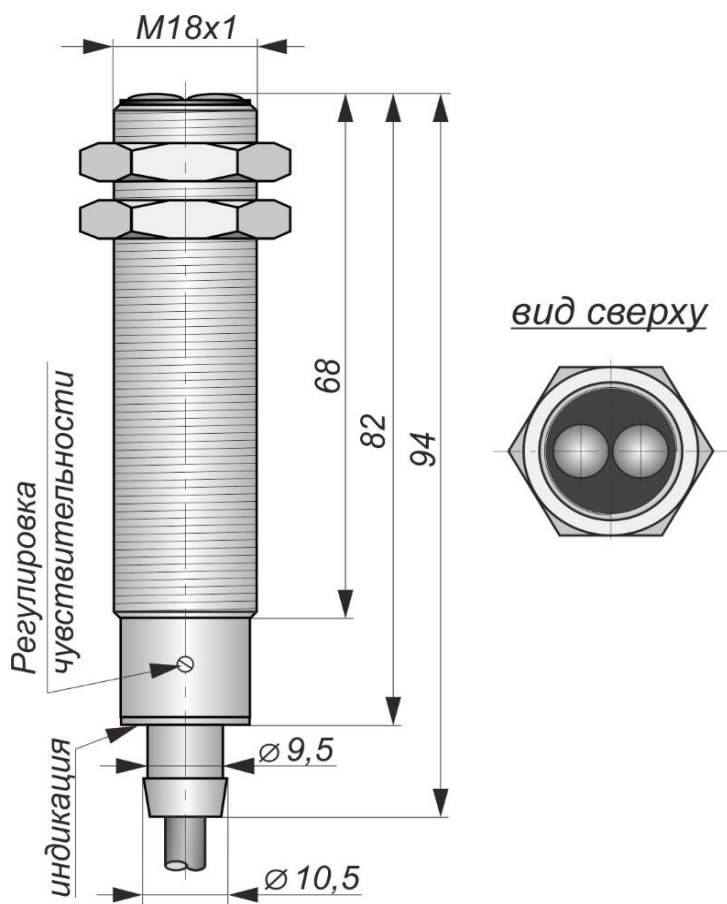
Габаритный чертеж
