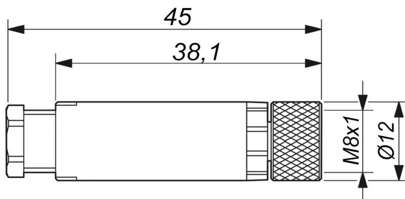
Габаритный чертеж
