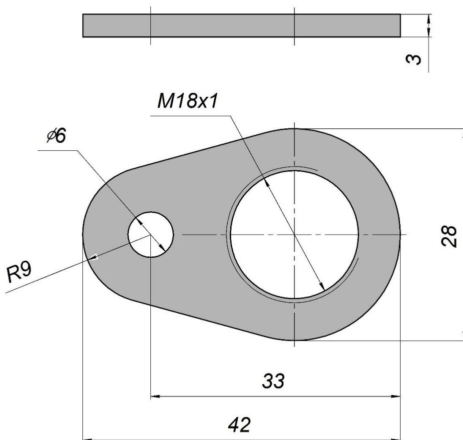
Габаритный чертеж
