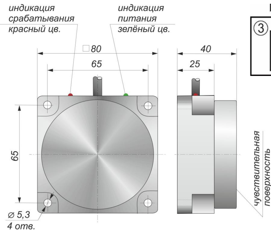
Габаритный чертеж
