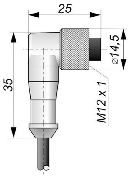
Габаритный чертеж
