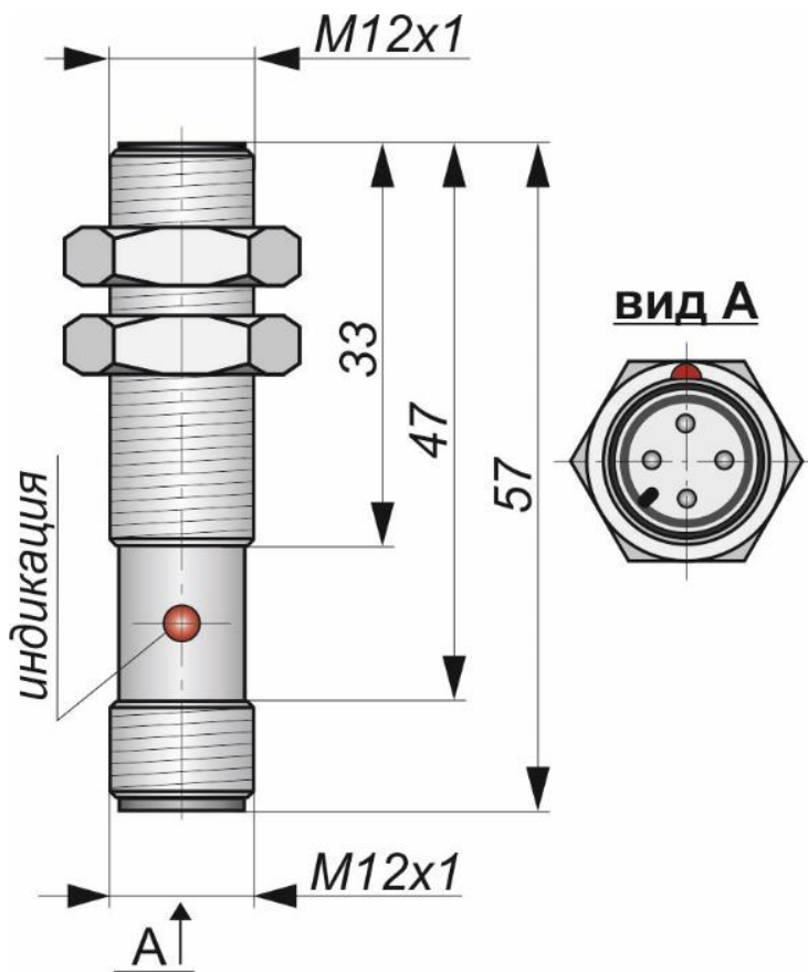
Габаритный чертеж
