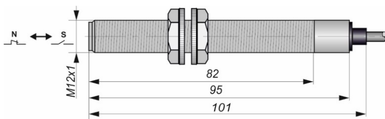
Габаритный чертеж
