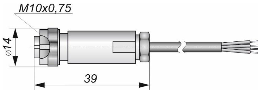
Габаритный чертеж
