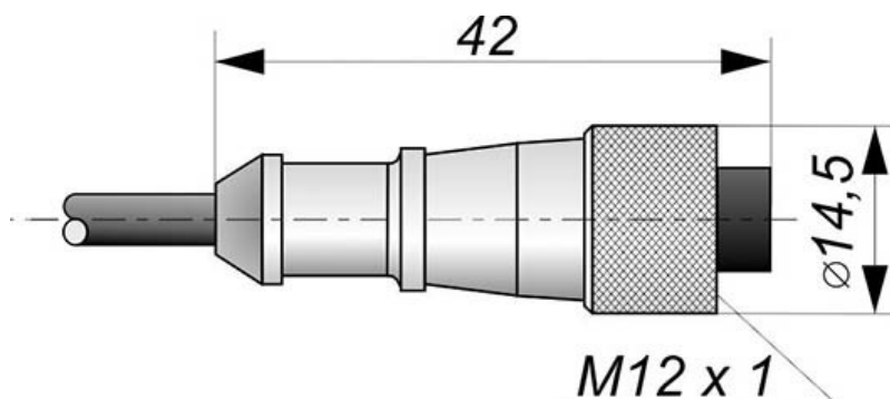
Габаритный чертеж
