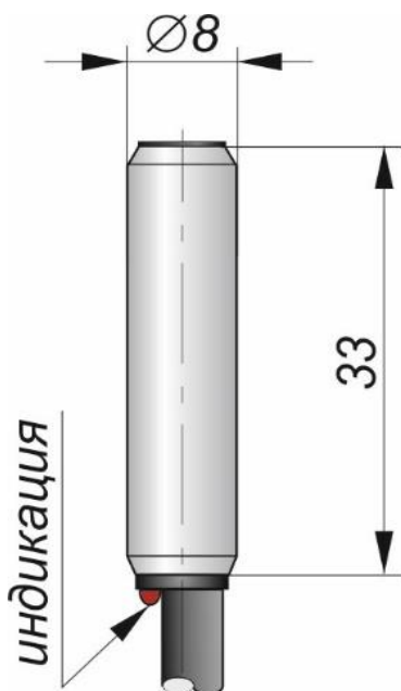
Габаритный чертеж
