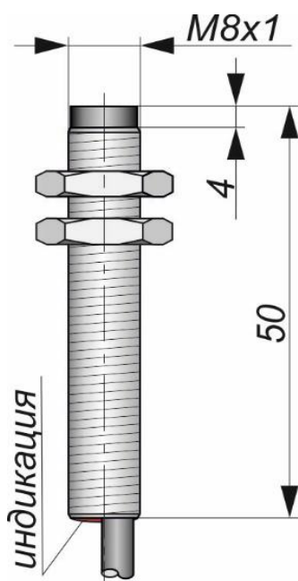
Габаритный чертеж
