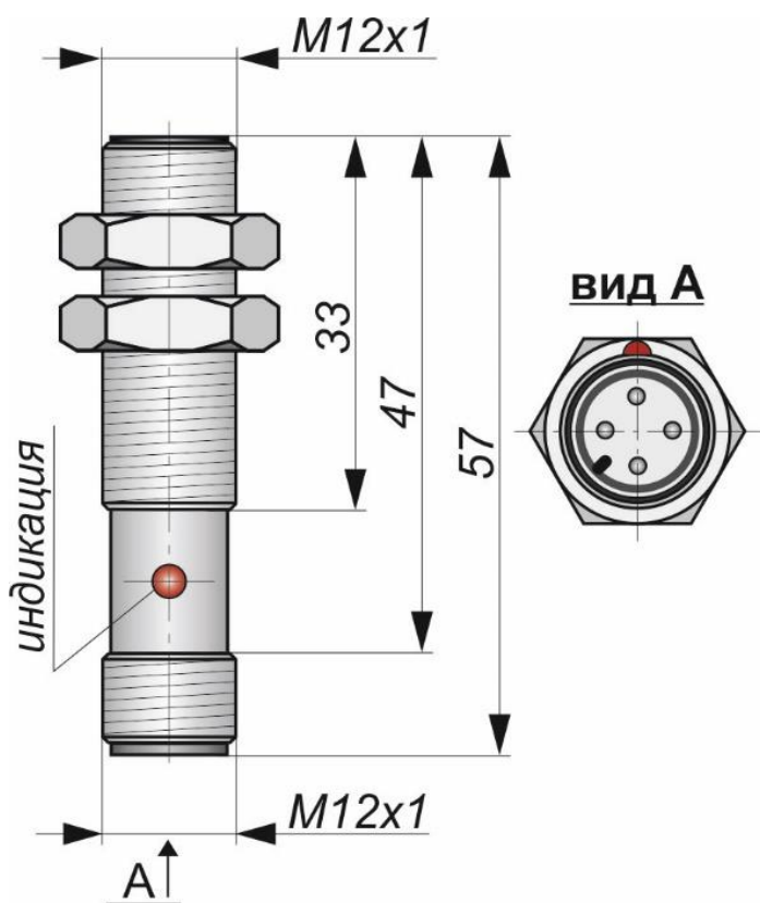
Габаритный чертеж
