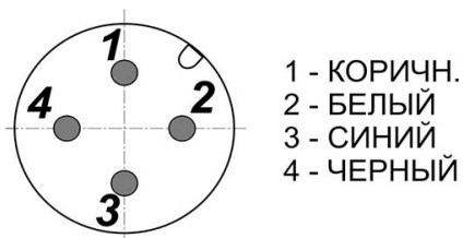
Цоколевка разъема
