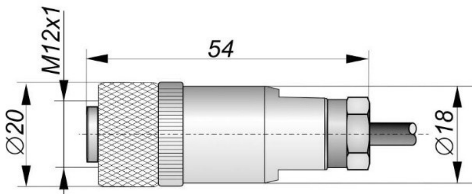
Габаритный чертеж
