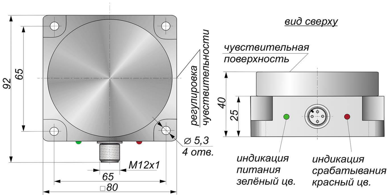
Габаритный чертеж
