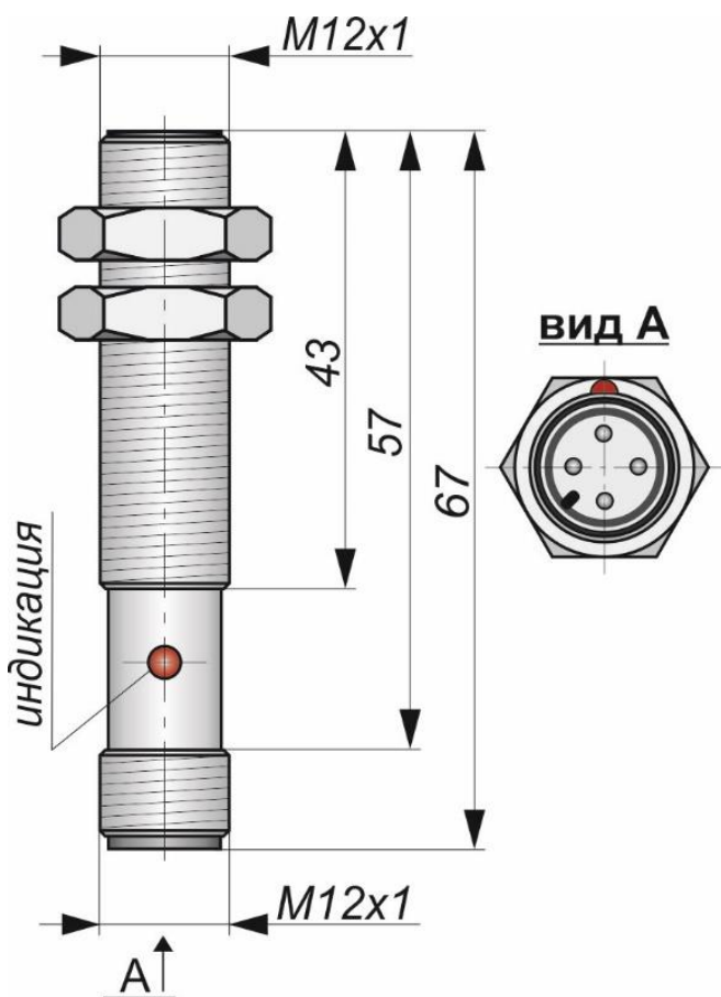
Габаритный чертеж
