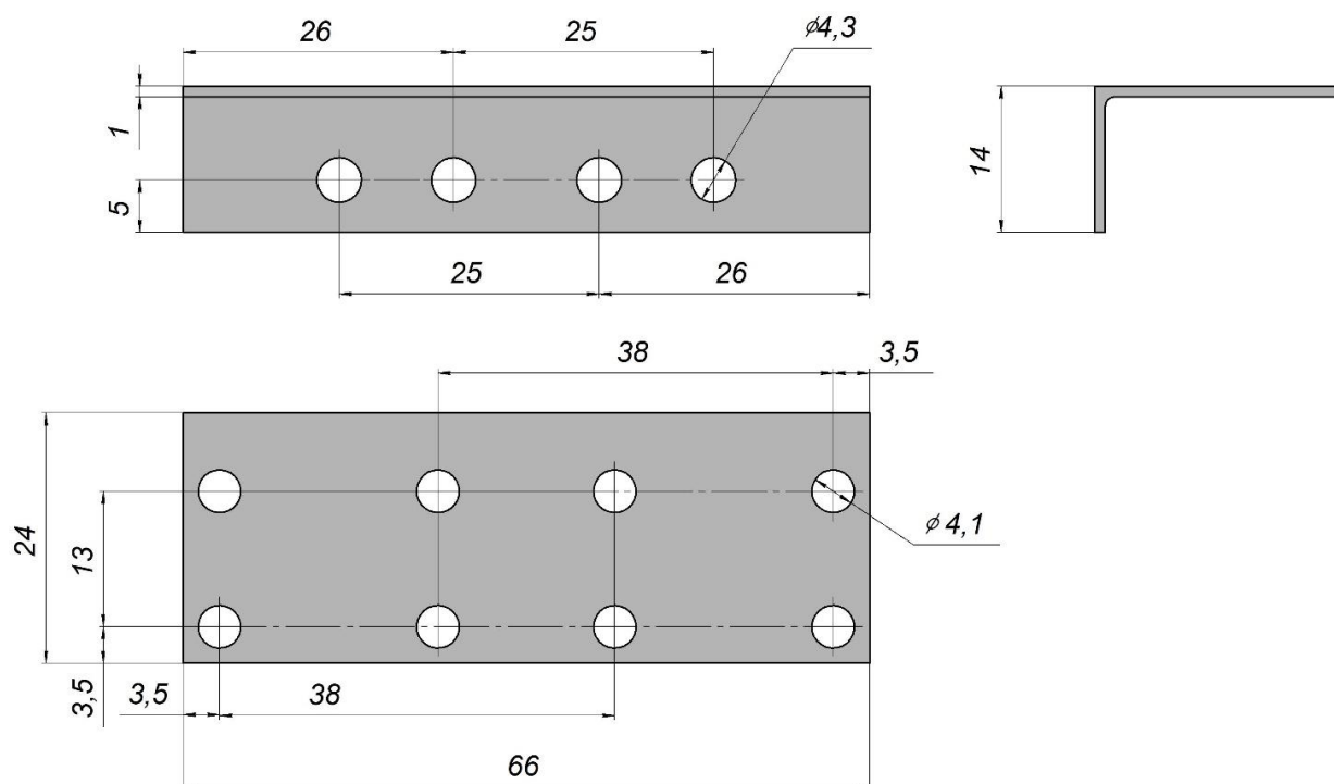
Габаритный чертеж
