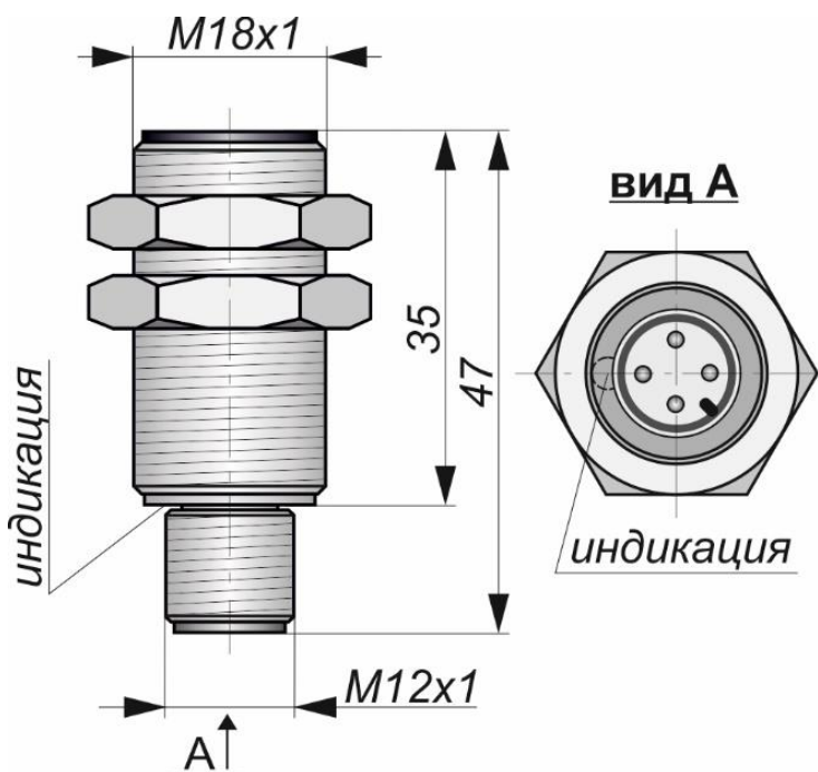
Габаритный чертеж
