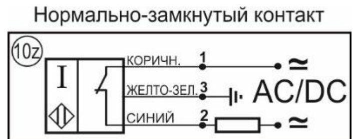
Схема соединения
