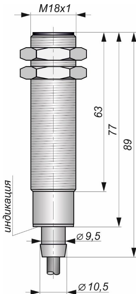
Габаритный чертеж
