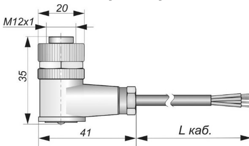
Габаритный чертеж
