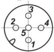
XS1(розетка)
