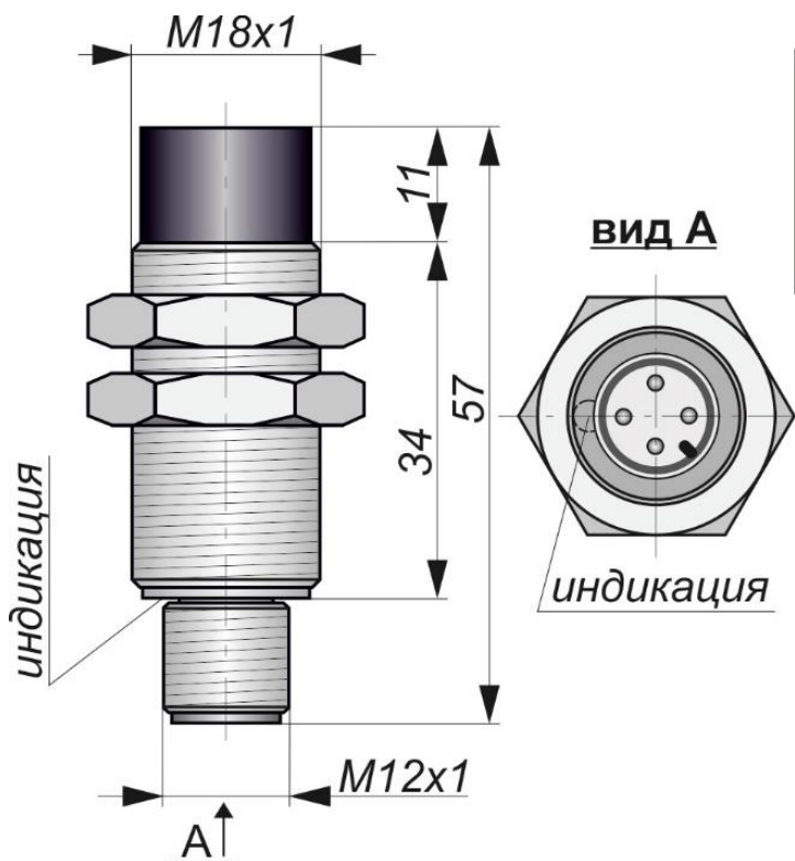
Габаритный чертеж
