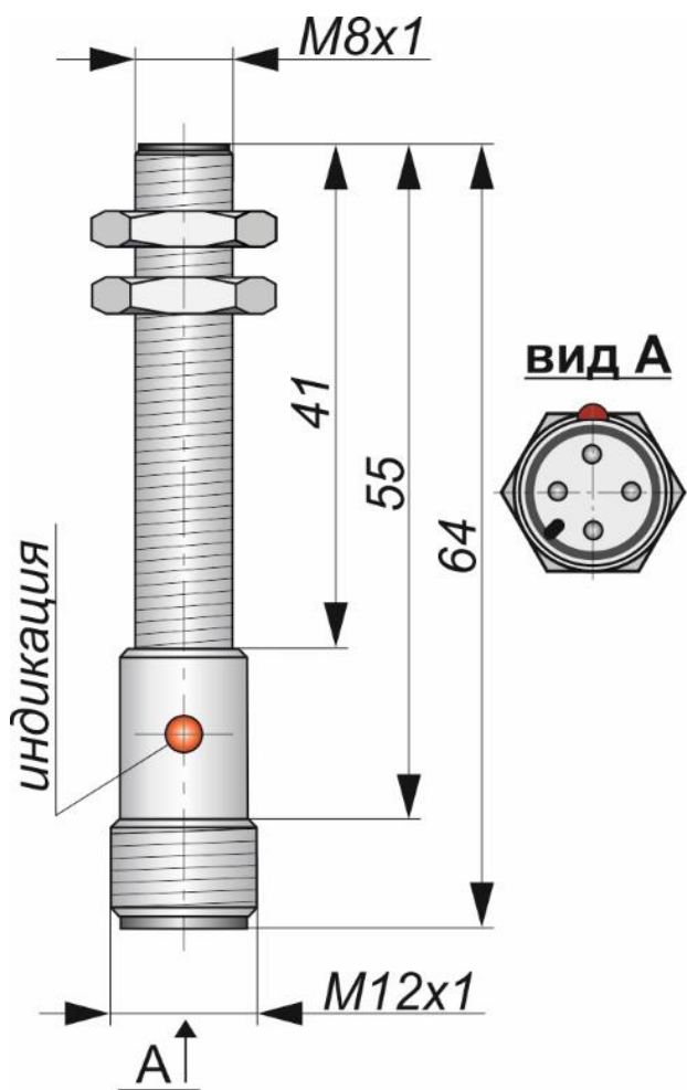
Габаритный чертеж
