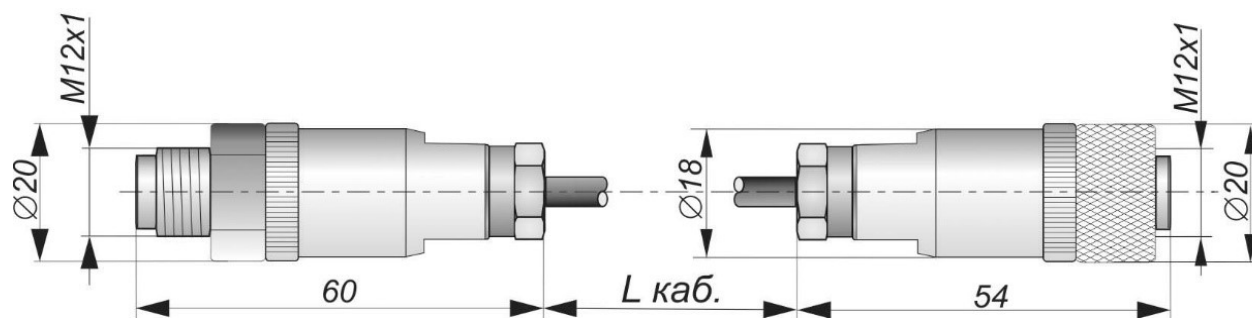
Габаритный чертеж
