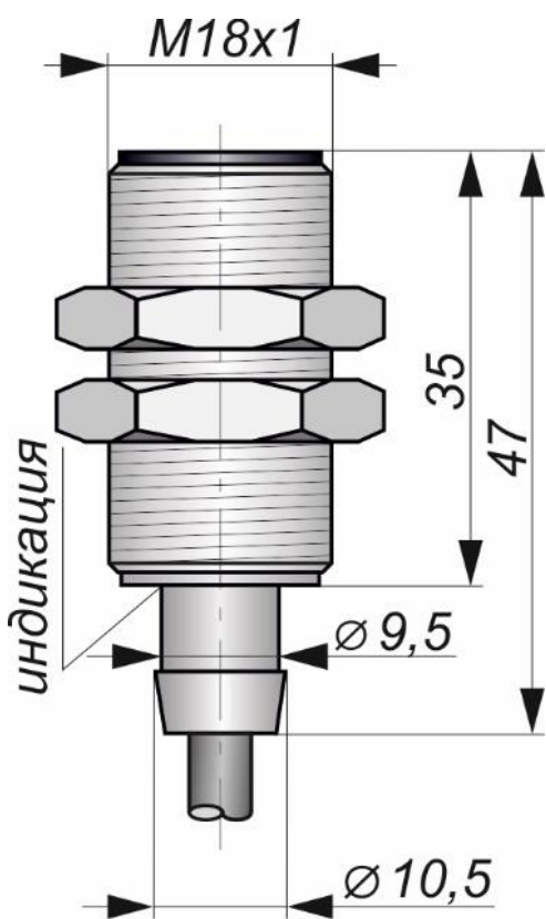
Габаритный чертеж
