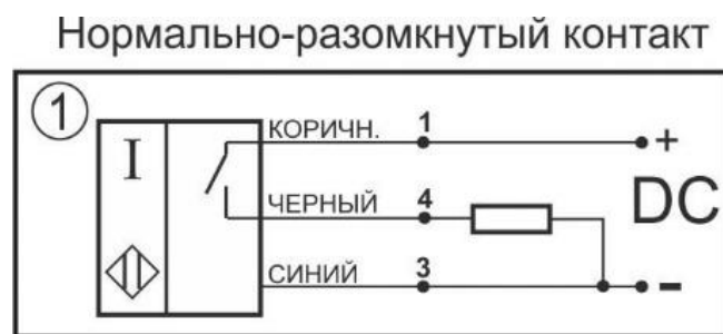
Схема соединения
