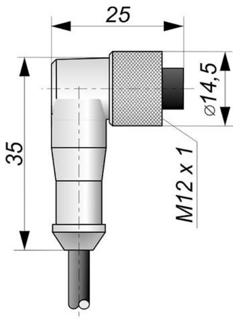
Габаритный чертеж
