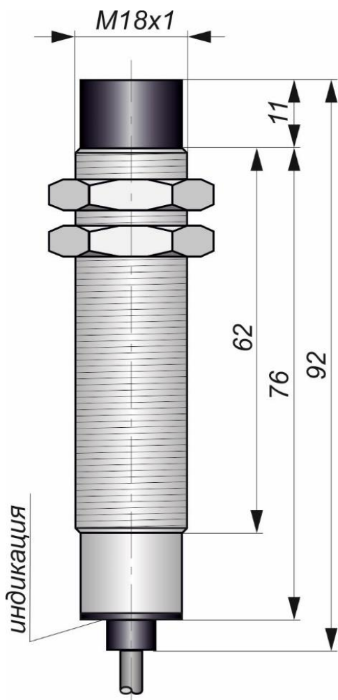
Габаритный чертеж
