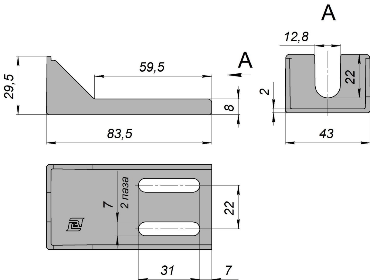
Габаритный чертеж
