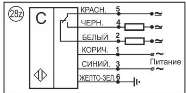
Схема соединения
