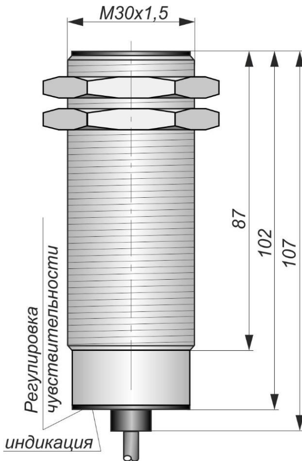
Габаритный чертеж
