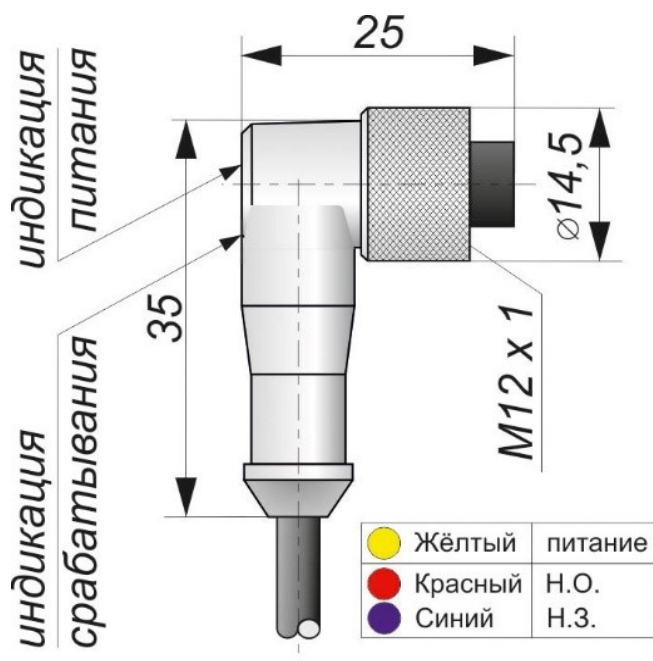
Габаритный чертеж
