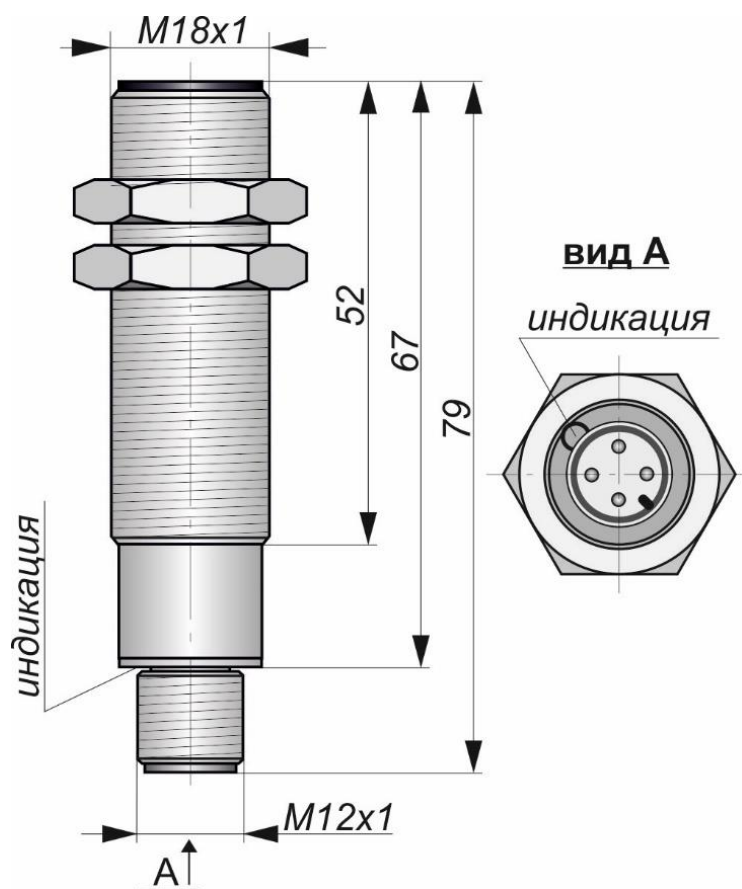
Габаритный чертеж
