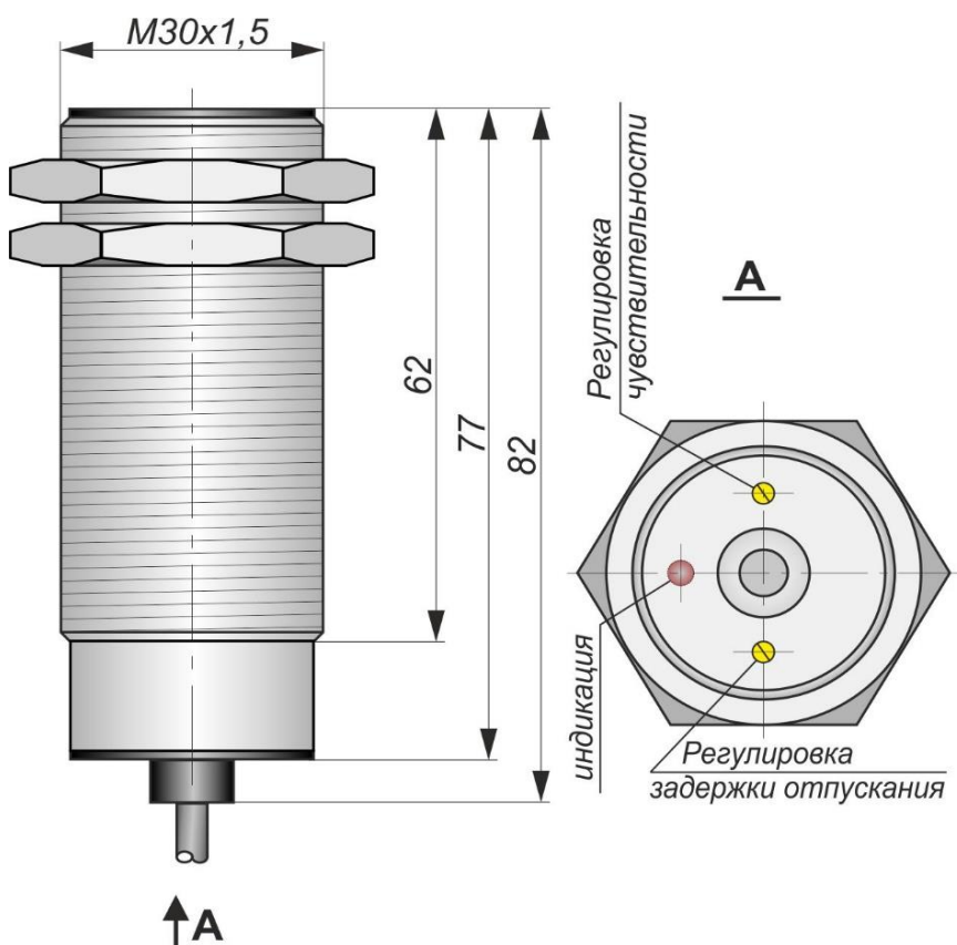
Габаритный чертеж
