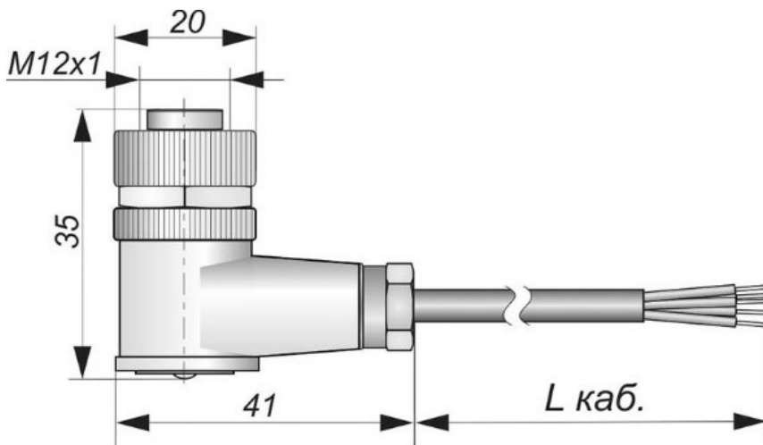
Габаритный чертеж
