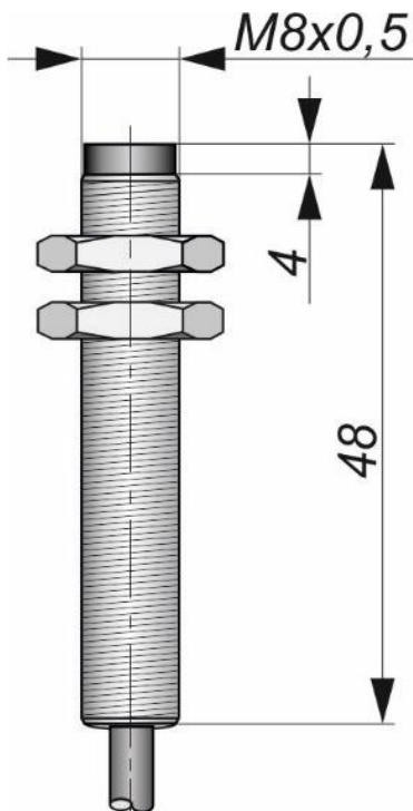
Габаритный чертеж
