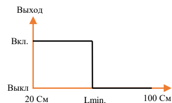
Рис. 1. Диаграмма работы выхода датчика модификации М1
