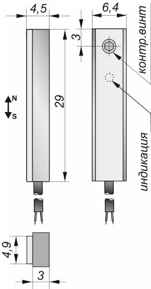
Габаритный чертеж
