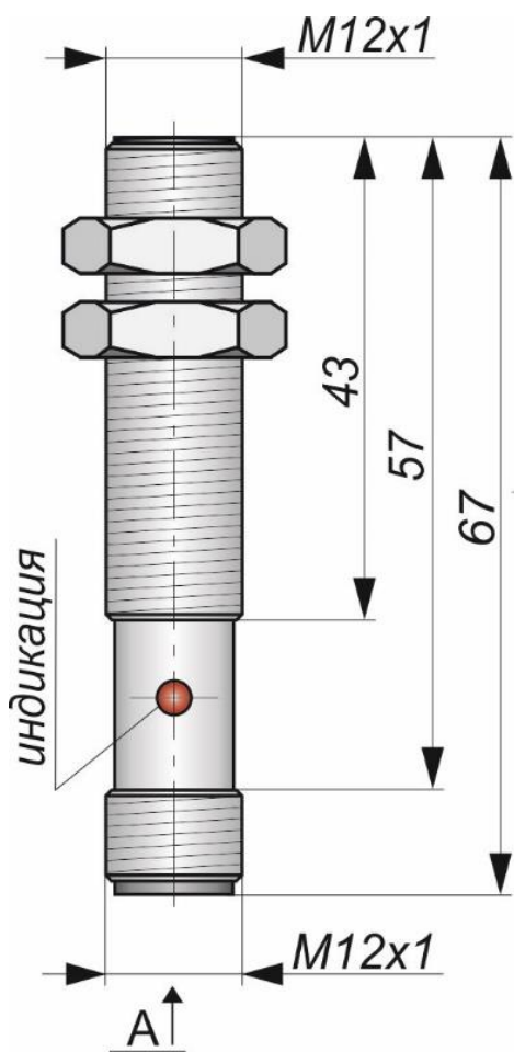
Габаритный чертеж
