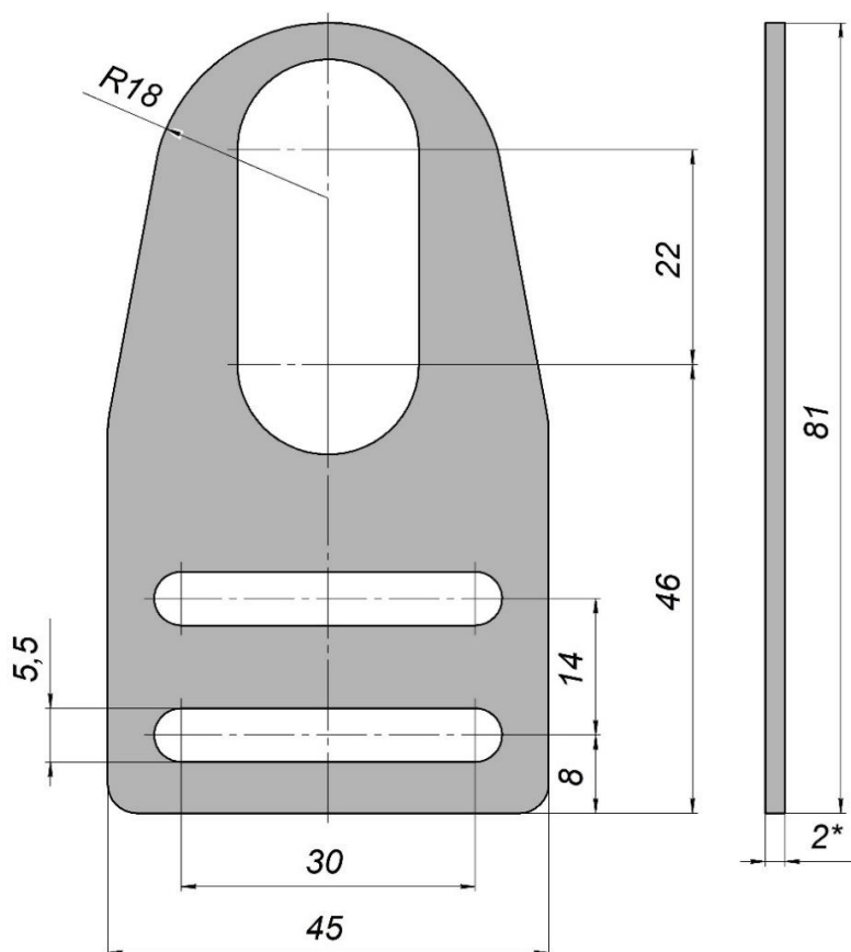
Габаритный чертеж
