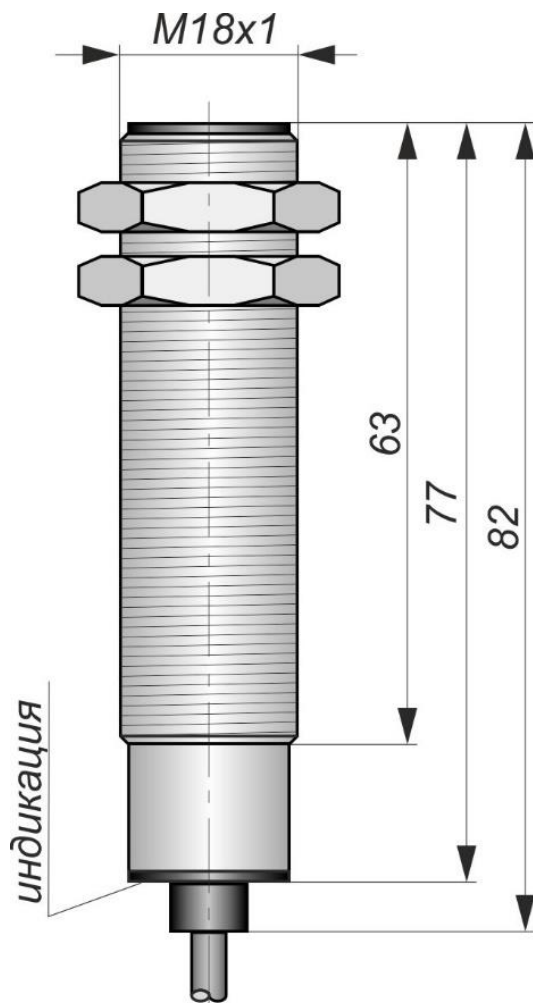
Габаритный чертеж
