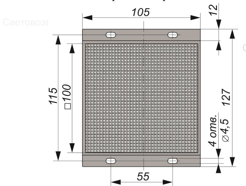
Габаритный чертеж
