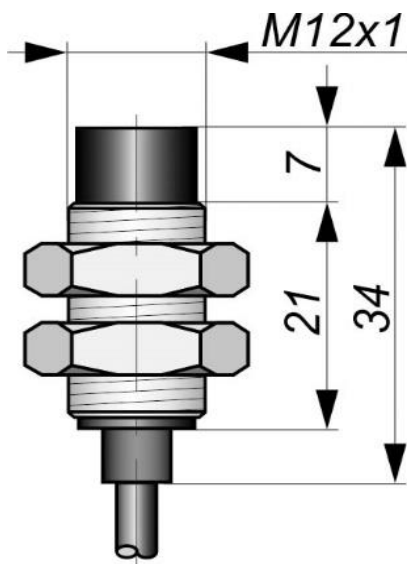
Габаритный чертеж
