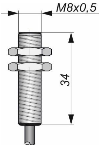
Габаритный чертеж
