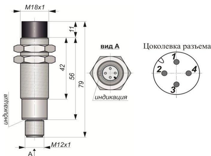
Габаритный чертеж
