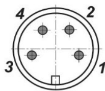
Цоколевка разъема
